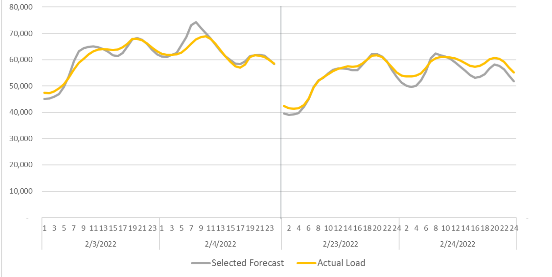
Load Forecast vs. Actual - 6 hour ahead
