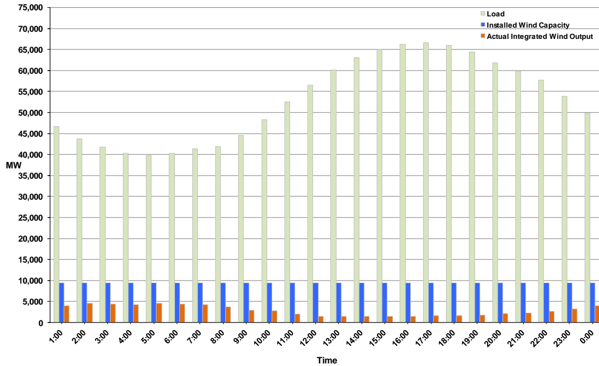
Hourly Average Actual Load vs. Actual Wind Output 08-05-2011
