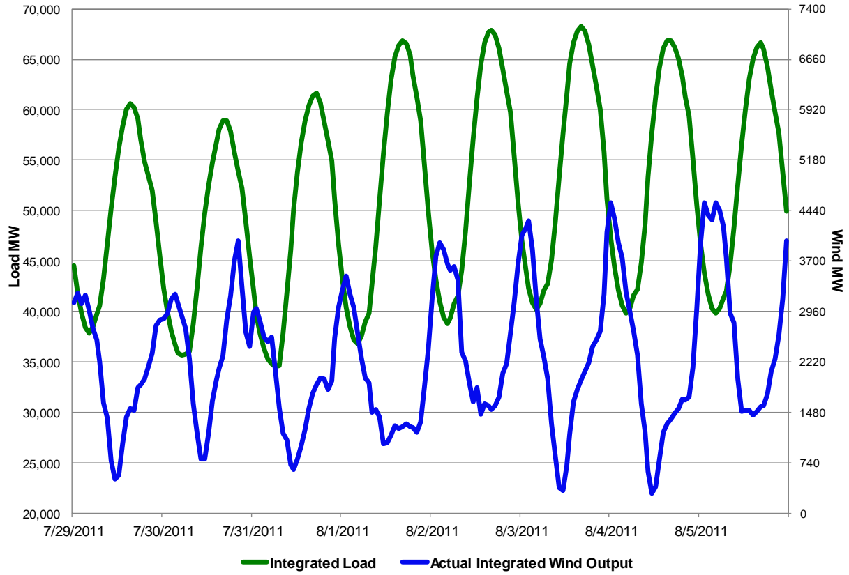
ERCOT Load vs. Actual Wind Output 7/29/2011 - 8/5/2011
